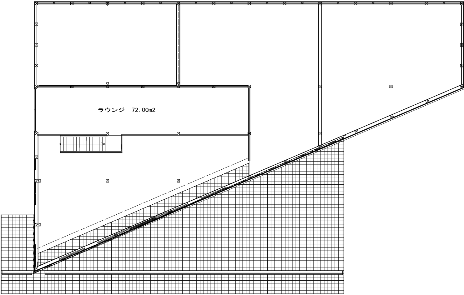
2階平面図
