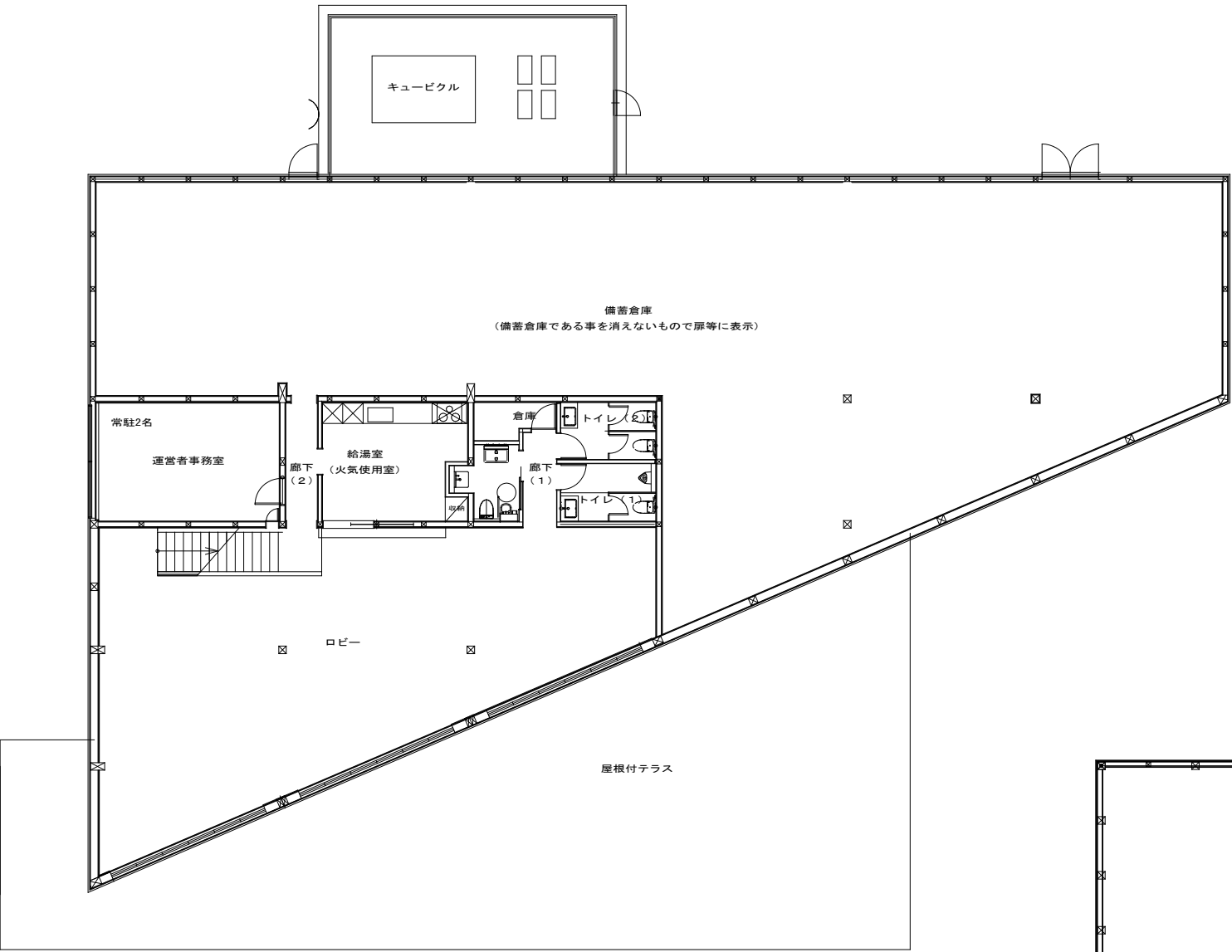
1階平面図
